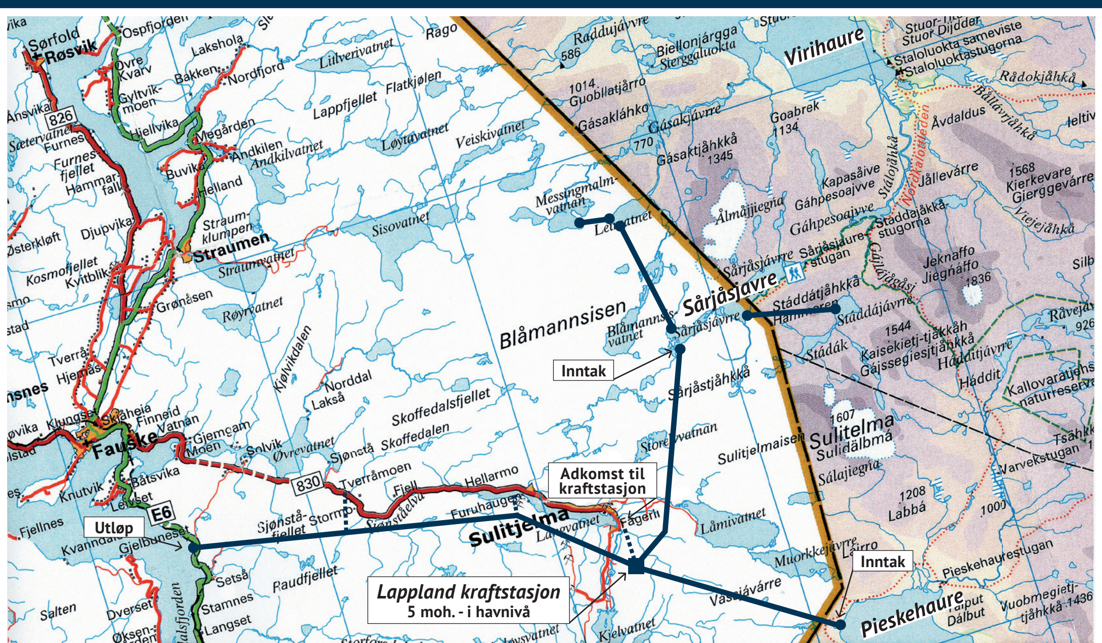
Bajep Sårjåsjavre (822 moh.) og Pieskehaure (577 moh.) reguleres til Lappland kraftstasjon (5 moh.) i Sulitelma.
